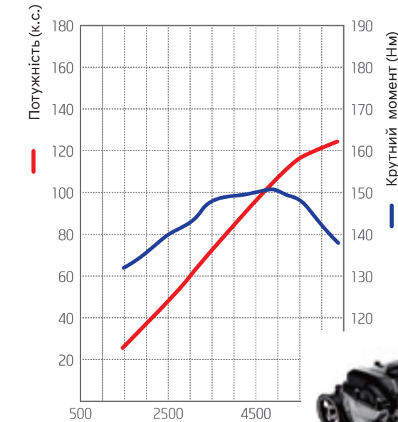
Двигун Gamma 1.6 D-CVVT
